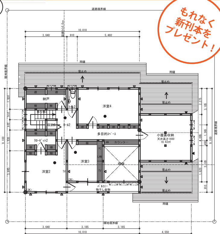
2階平面図
