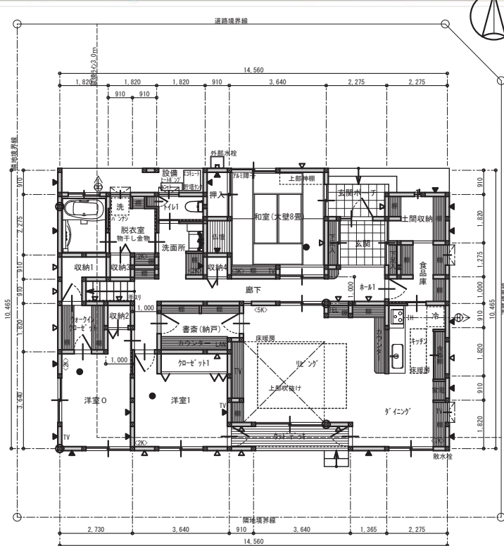
1階平面図
